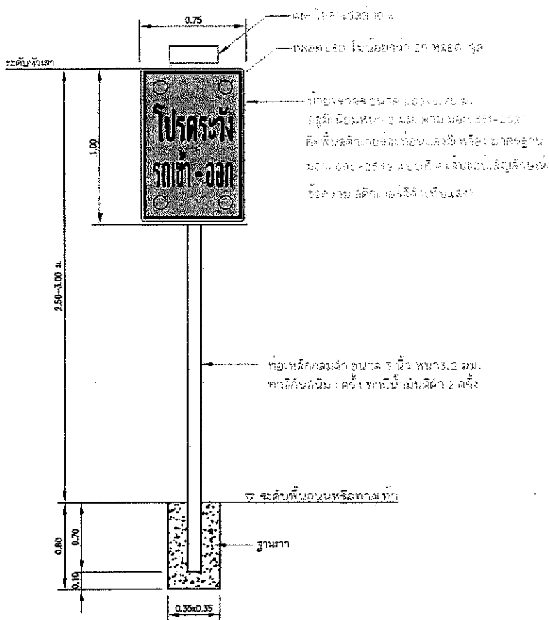
แบบที่ ๒ ระวังรถเข้า-ออก เขตปรับปรุงผิวจราจร
