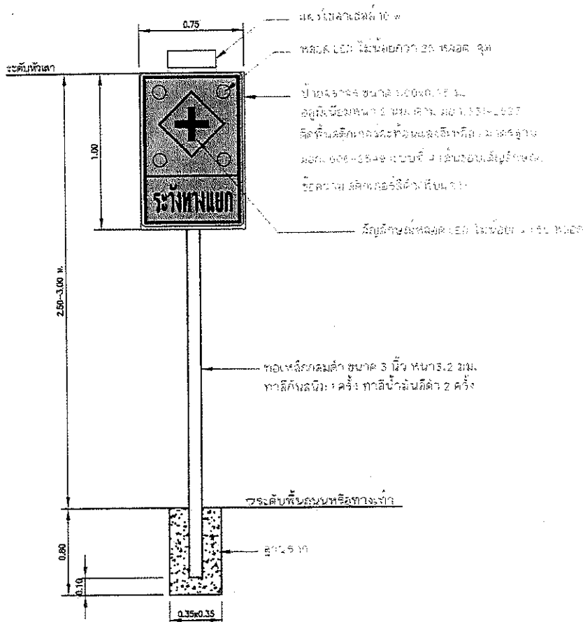
แบบที่ ๑ ระวังคนชก ทางเขตโครงการปรับปรุงผิวจราจร
