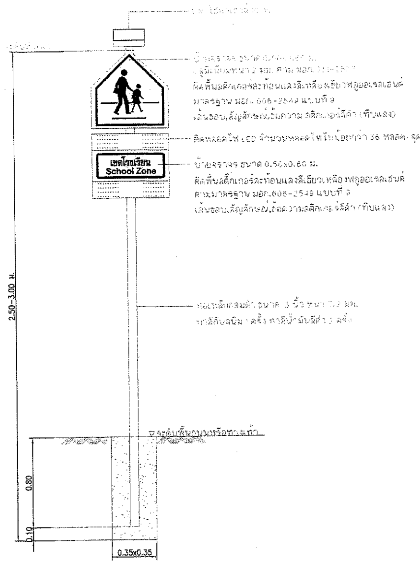
แบบที่ 5 ป้ายเตือนเขตโรงเรียน ไฟกระพริบโซล่าเซลล์
