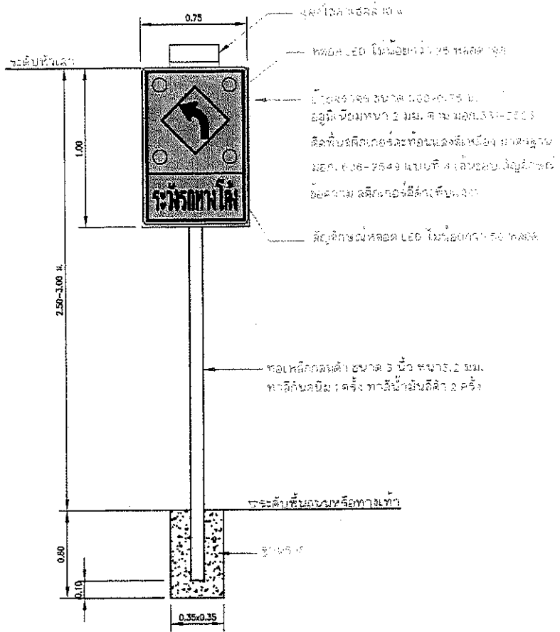
แบบที่ 1 ป้ายเตือนการหักซ้าย ไฟกระพริบโซล่าเซลล์
