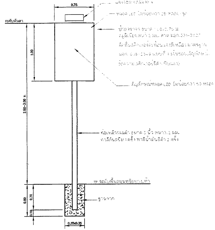
แบบที่ 2 ป้ายเตือนการหักขวา ไฟกระพริบโซล่าเซลล์
