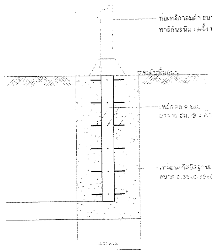
แบบขยายฐานราก ①
