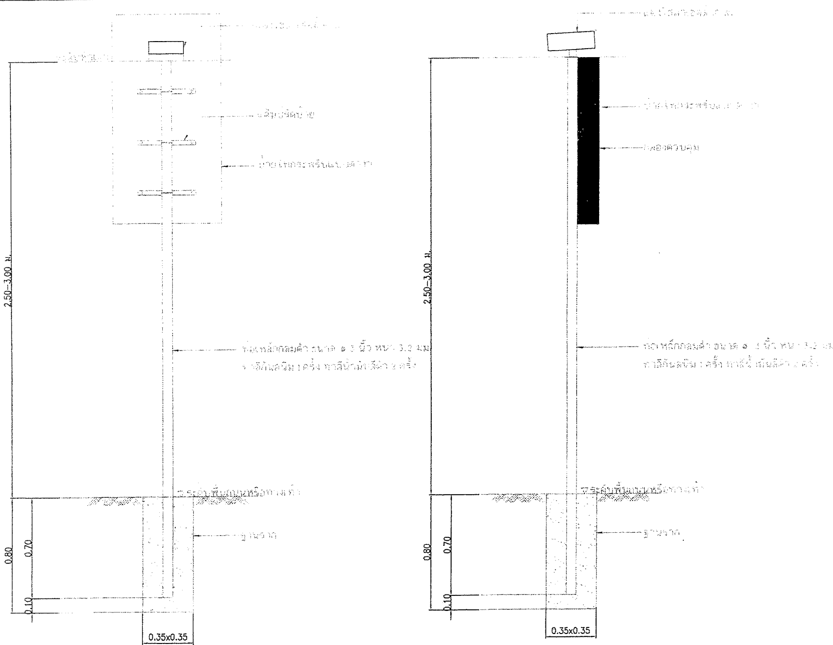
รูปแบบด้านหลัง - ด้านข้าง บ้ายไฟกระพริบโซล่าเซลล์ 1,2,3 และ 4
