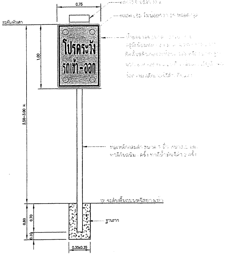
รูปที่ 1.11 - ป้ายจราจรเตือนภัย (โปรดระวังรถเข้า-ออก)
