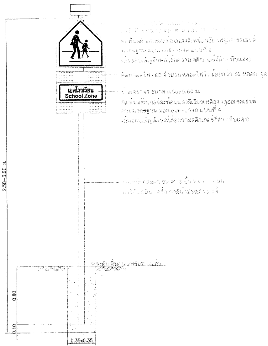
แบบที่ 5 ป้ายเตือนเขตโรงเรียน ไฟกระพริบโซล่าเซลล์
