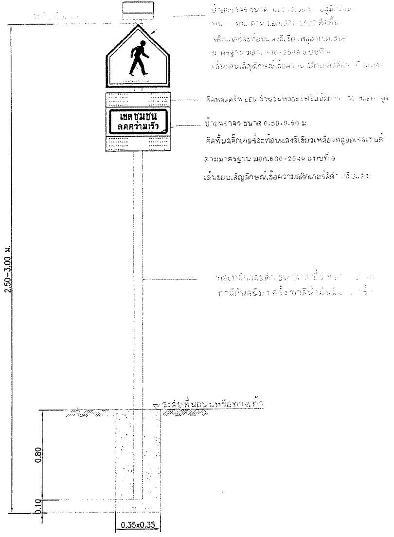
แบบที่ 6 ป้ายเตือนเขตชุมชนลดความเร็ว ไฟกระพริบโซล่าเซลล์
