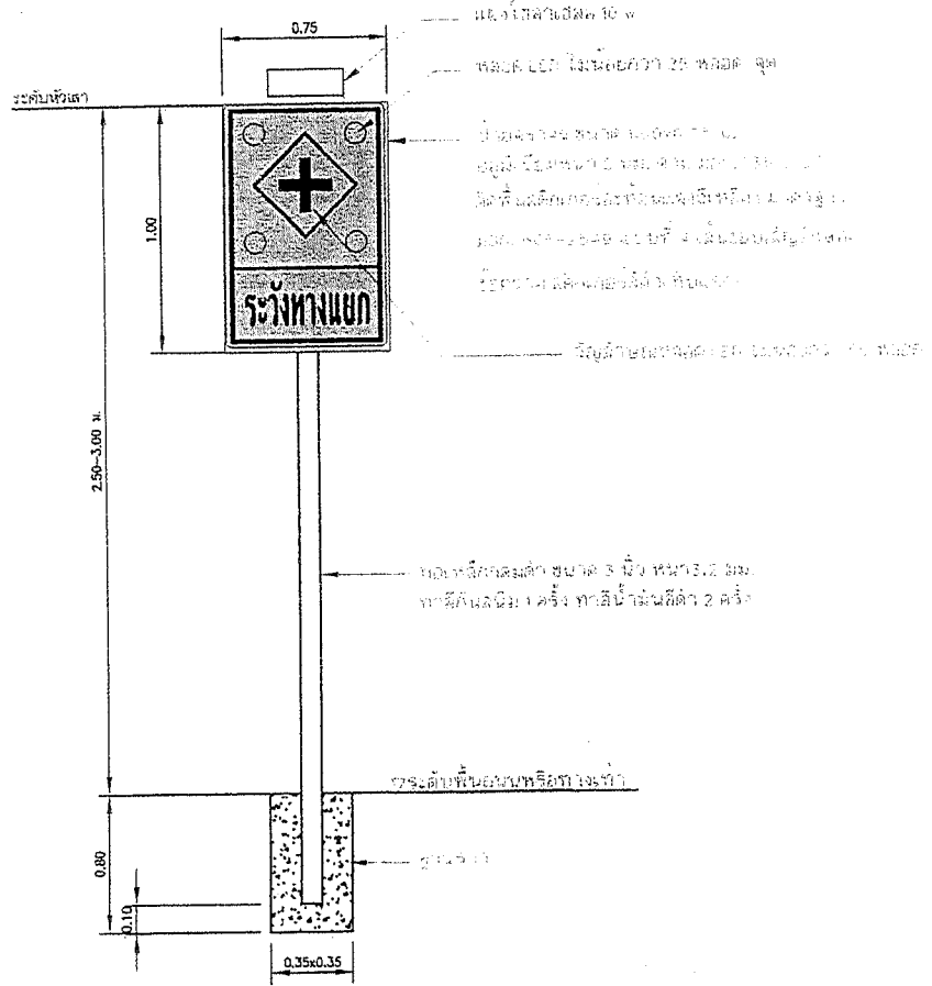
รูปที่ 1.10 - ป้ายจราจรเตือนภัย (ระวังทางแยก)
