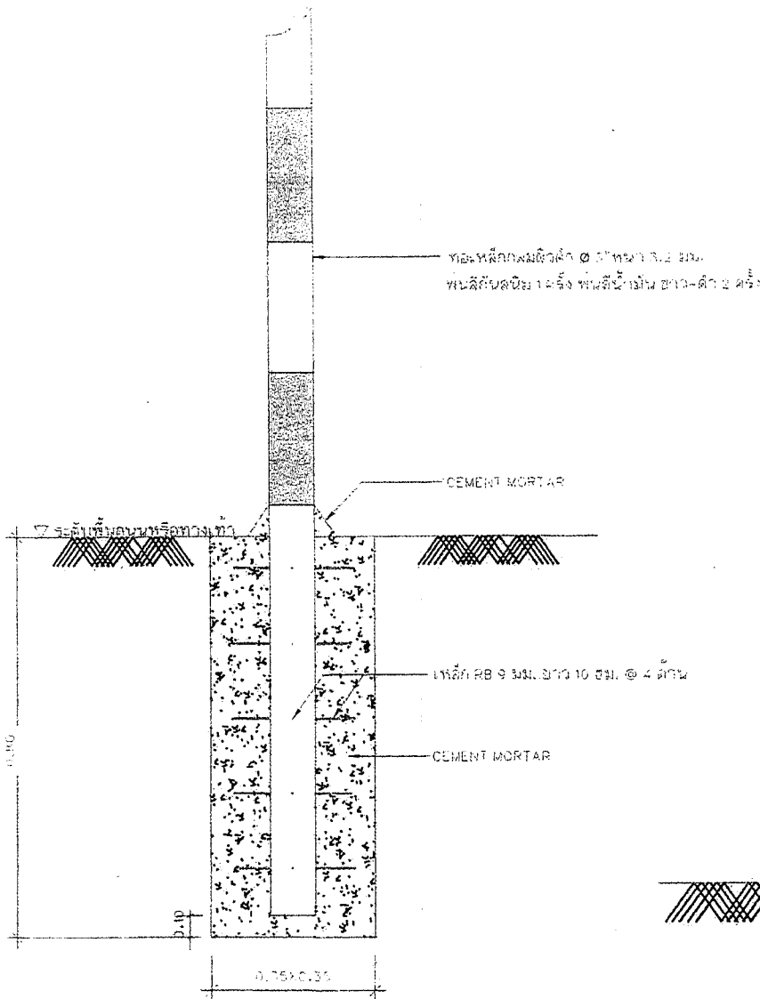
แบบขยายฐานจาก ①
