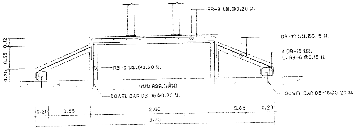
แบบขยายฐานราก (ป้ายชื่ออาคาร)
