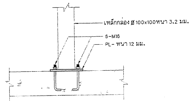
แบบขยายการติดตั้งเสาป้ายชื่ออาคาร
