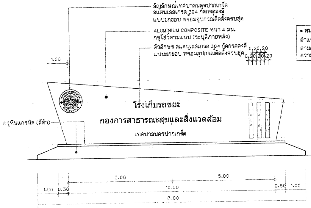
รูปด้าน-1 (ป้ายชื่ออาคาร) SCALE 1:75
