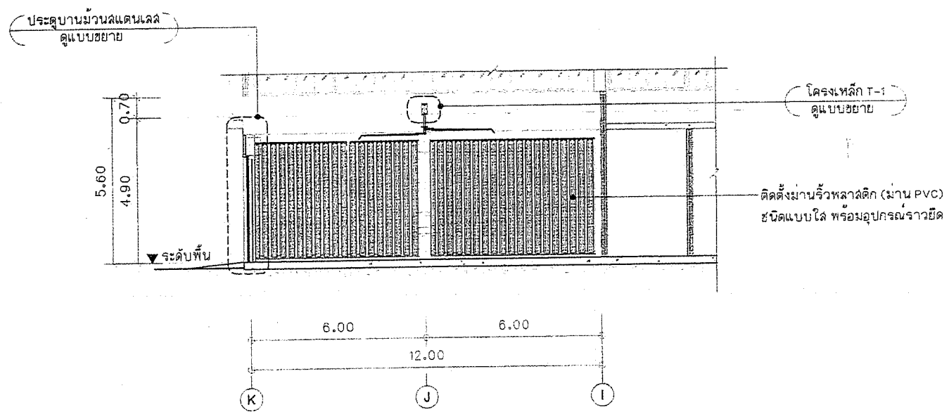
รูปตัด-B (ระบปล่างจรด) SCALE 1:125
