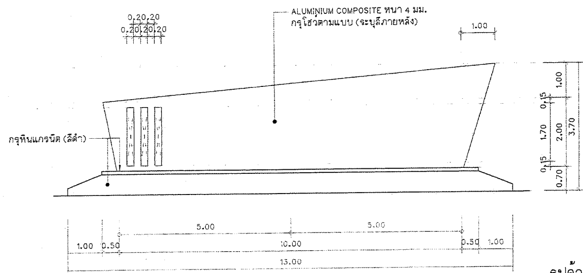
รูปด้าน-2 (ป้ายชื่ออาคาร) SCALE 1:75
