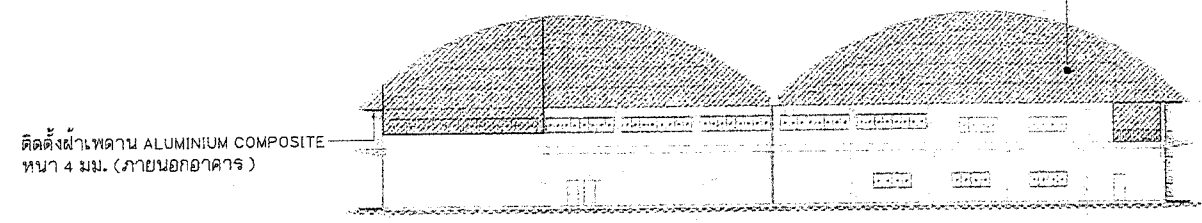
รูปตัด-A (ติดตั้งตาข่ายกันนก HDPE) SCALE 1:400
