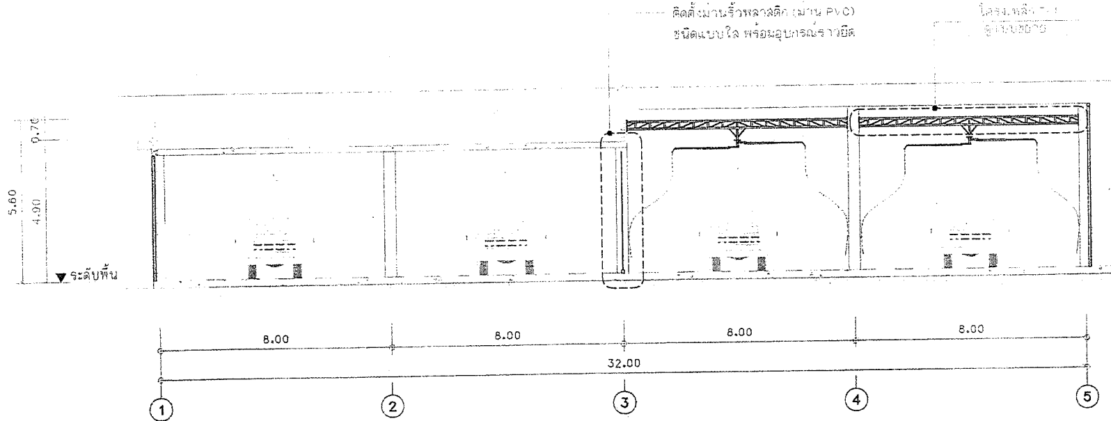
รูปตัด-A (ระบปล่างจรด) SCALE 1:125
