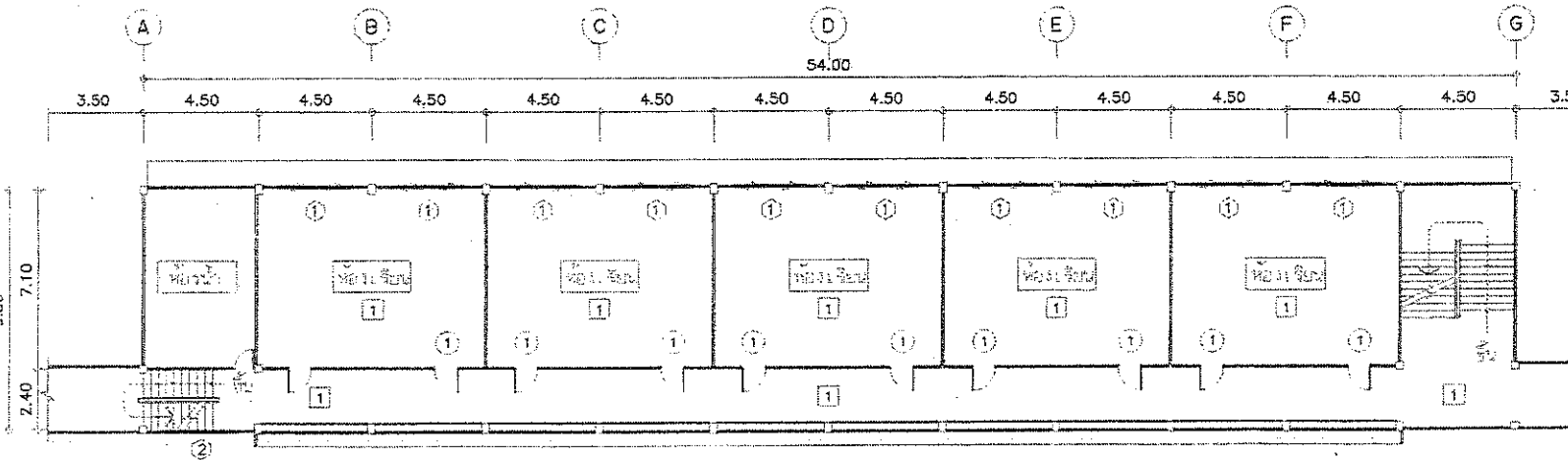
แปลนพื้นที่ 1 (อาคารพุทธรักษา) SCALE 1:200
