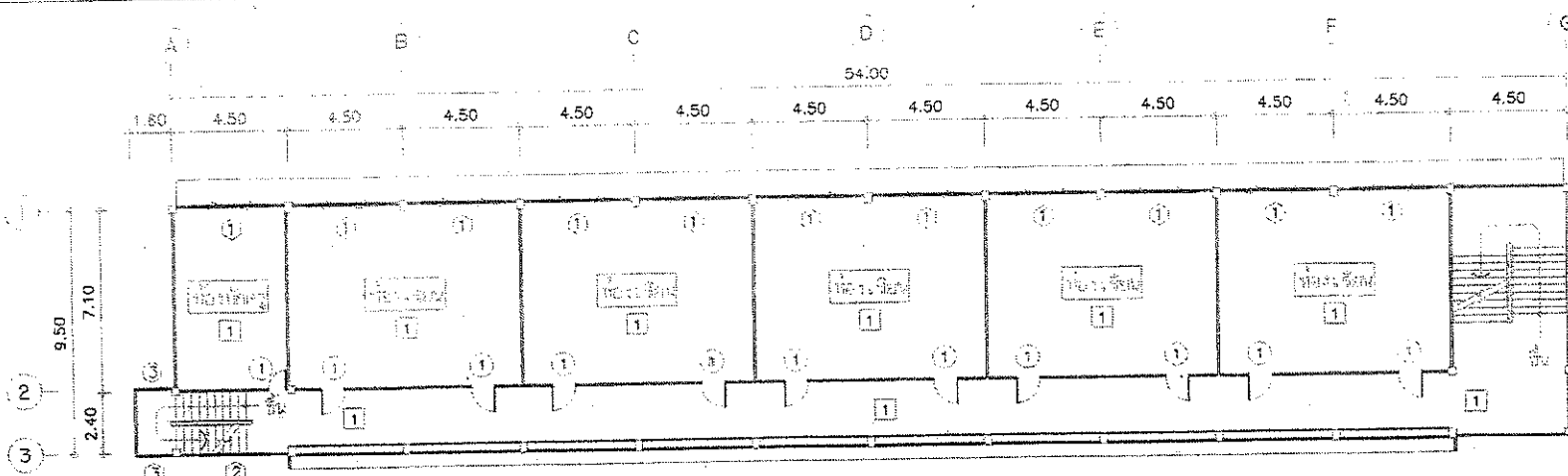
แปลนพื้นที่ 3 (อาคารพหุศึกษารักษา) SCALE 1:200
