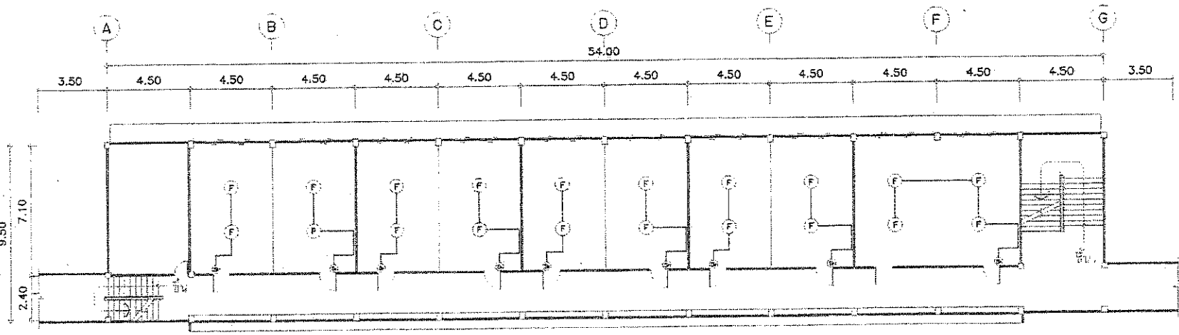
แปลนรูปตัดลมและติดตั้งพัดลมชั้นที่ 1 (อาคารฟิสิกส์) SCALE 1:200
