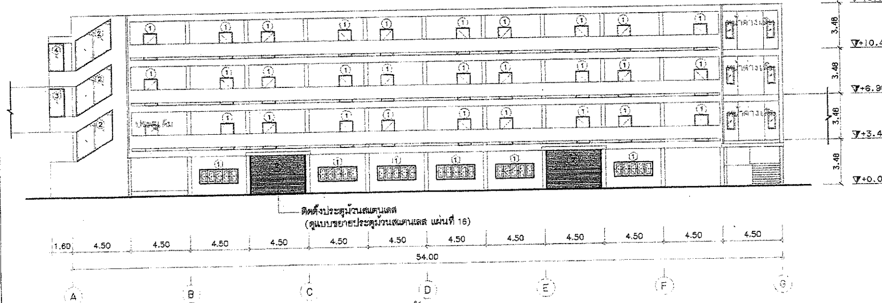
รูปด้าน - 1 SCALE 1:200
