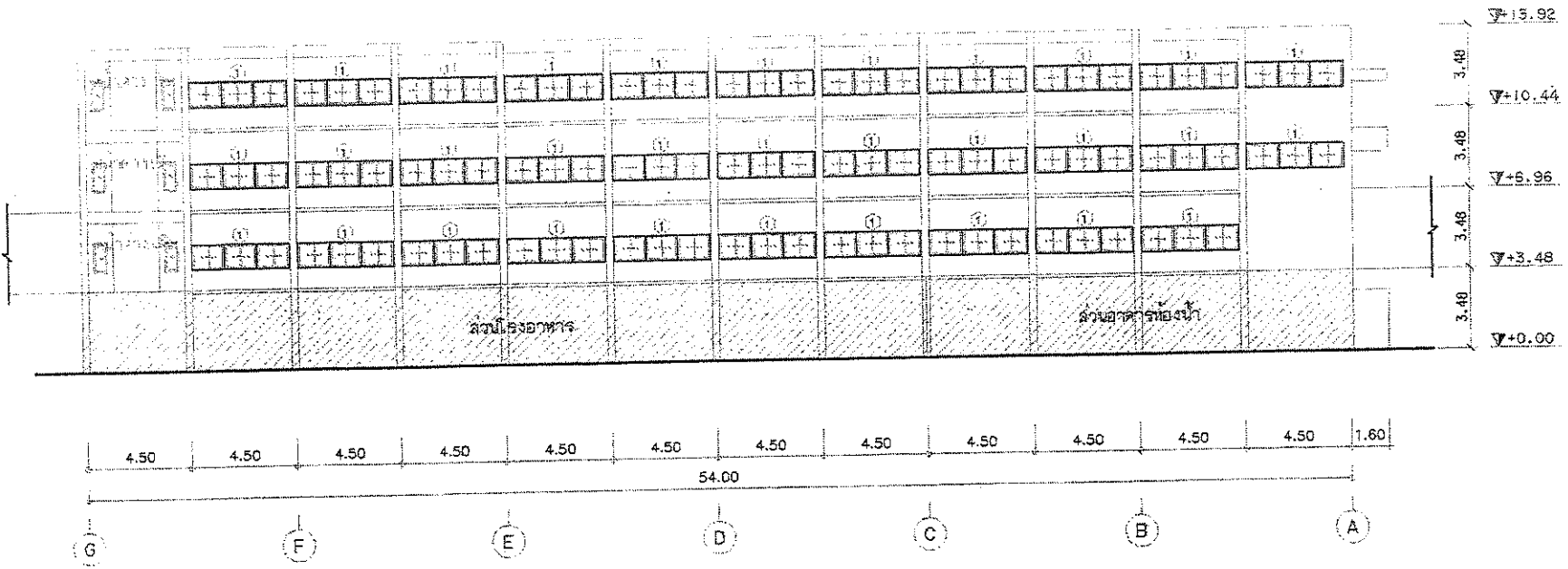
รูปด้าน - 3 SCALE 1:200
