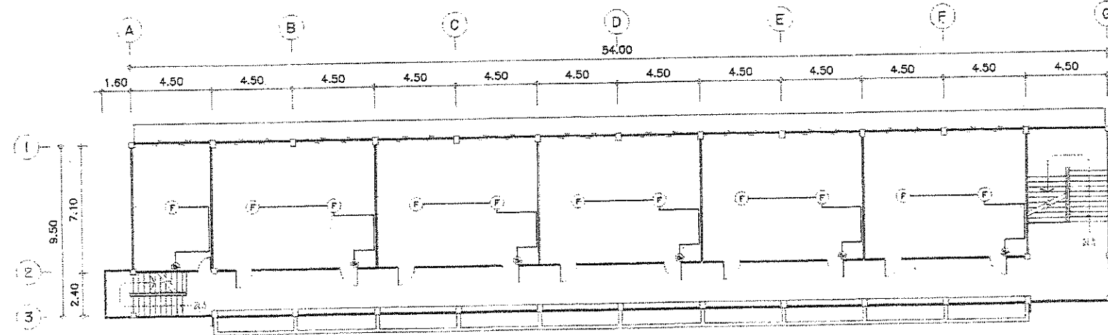
แปลนรีดฝ้าและติดตั้งฝ้าลมชั้นที่ 3 (อาคารพุทธรักษา) SCALE 1:200
