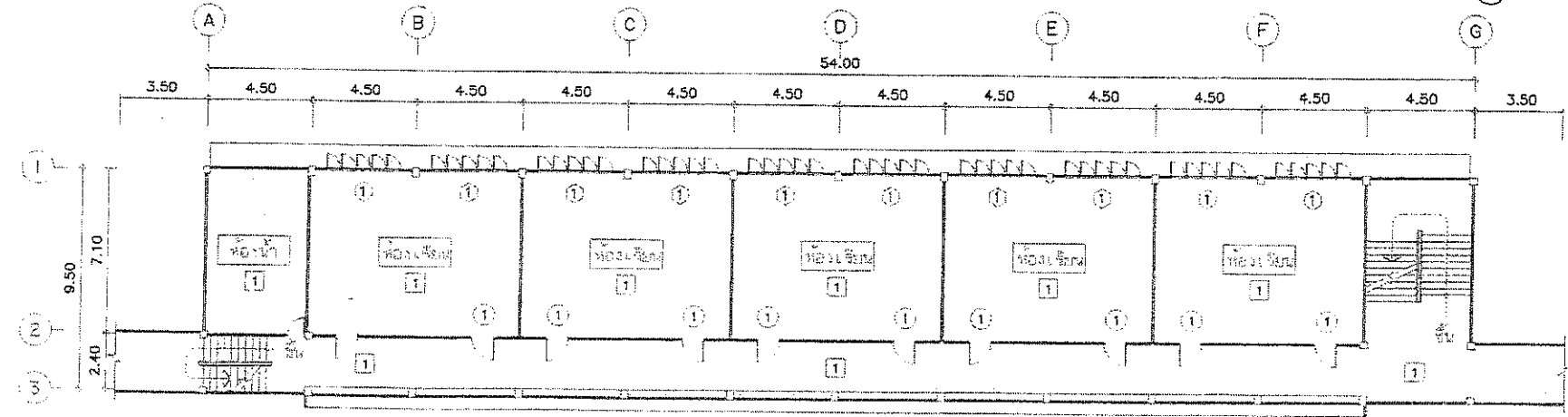
แปลนรีดถอนปรับปรุงชั้นที่ 1 (อาคารพุทธรักษา) SCALE 1:200
