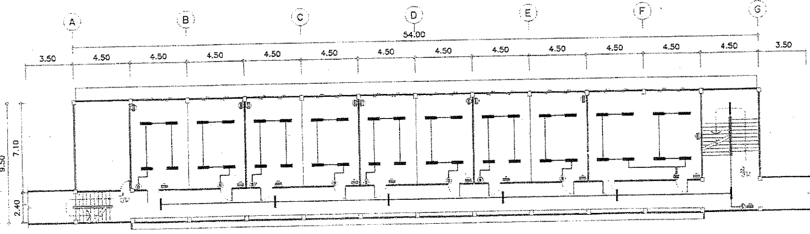
แปลนหรือระบบไฟฟ้าและติดตั้งระบบไฟฟ้าชั้นที่ 1 (อาคารพหุภักดิ์) SCALE 1:200
