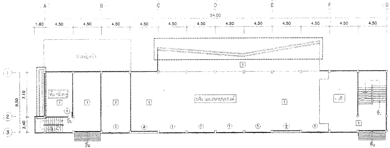
แปลนพื้นที่ 1 (อาคารพุทธรักษา) SCALE 1:200
