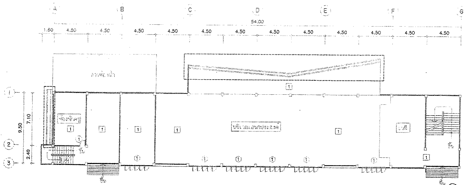
แปลนรีดถอนปรับปรุงชั้นที่ 1 (อาคารพุทธรักษา) SCALE 1:200
