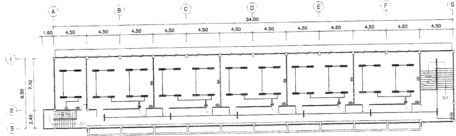
แผนรื้อระบบไฟฟ้าและติดตั้งระบบไฟฟ้าชั้นที่ 3 (อาคารพุดธิศึกษา) SCALE 1:200
