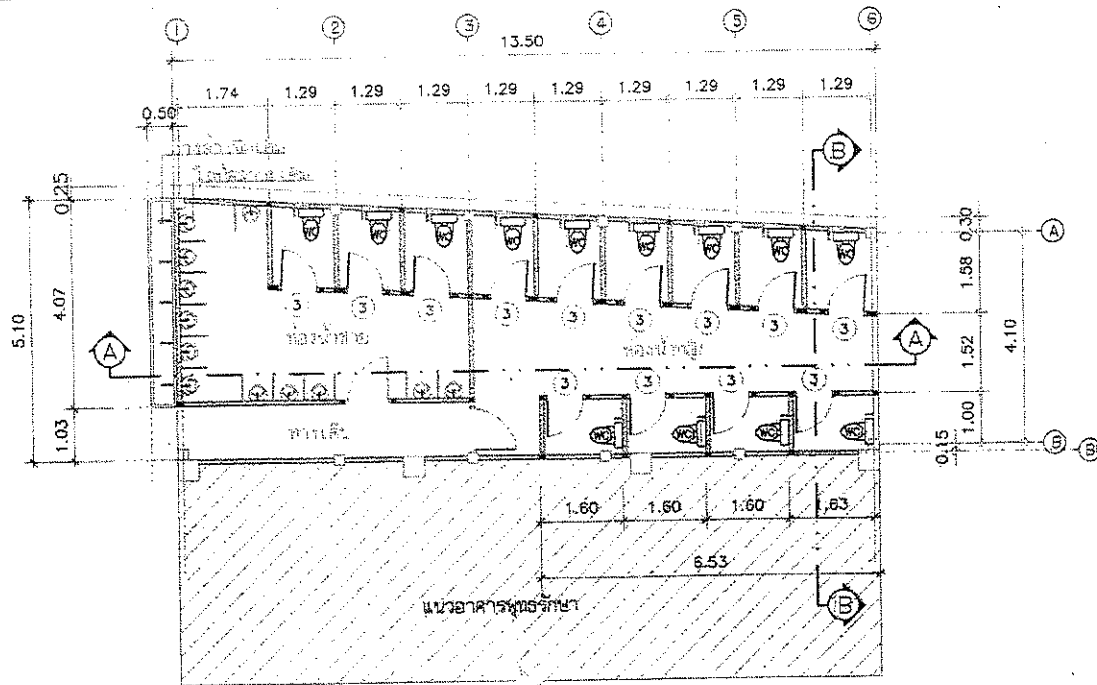
แปลนห้องน้ำ (หลังอาคารพุทธจริษา) SCALE 1:100
