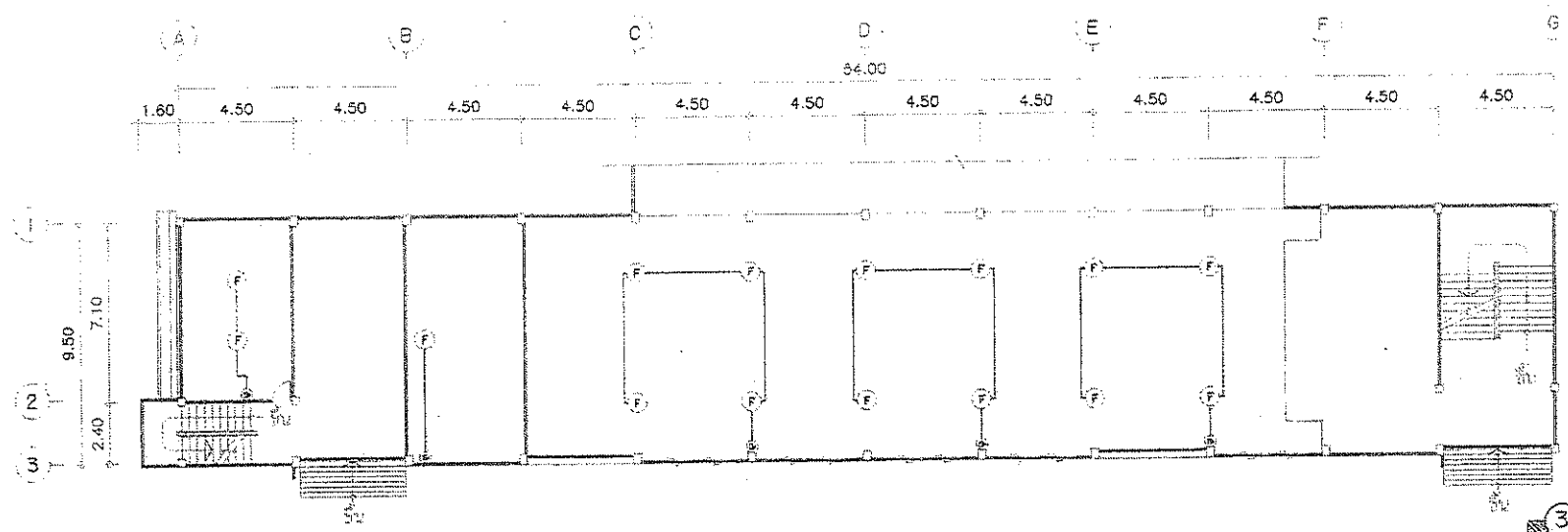
แปลนรูปตัดลมและติดตั้งพัดลมชั้นที่ 1 (อาคารฟิสิกส์) SCALE 1:200
