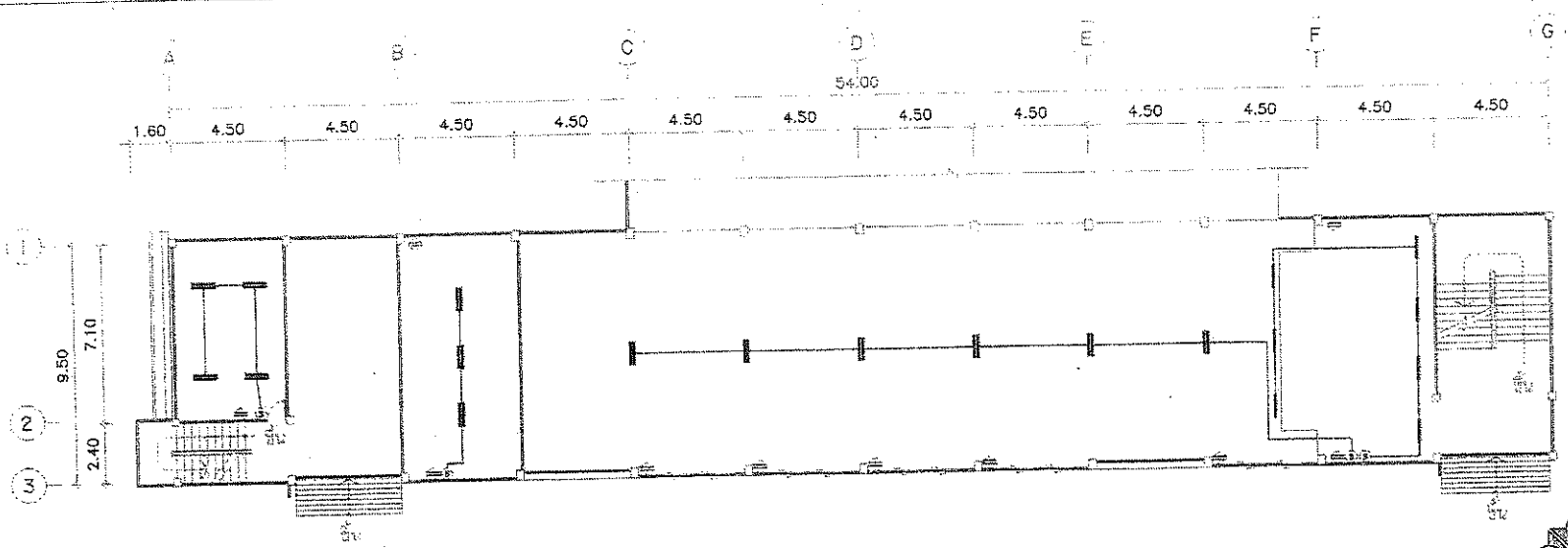
แปลนหรือระบบไฟฟ้าและติดตั้งระบบไฟฟ้าชั้นที่ 1 (อาคารพหุภักดิ์) SCALE 1:200
