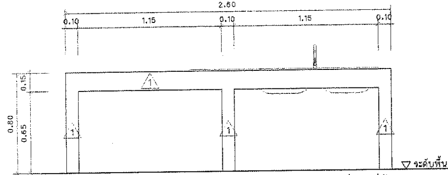
รูปด้าน (หน้า) เคาน์เตอร์ล้างจาน SCALE 1:20
