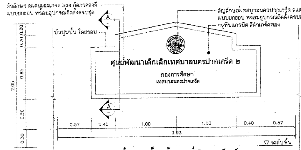
รูปด้าน (หน้า) ป้ายศูนย์พัฒนาเด็กเล็ก SCALE 1:25
