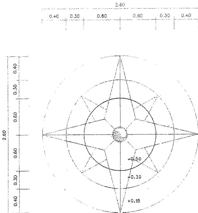
แปลนพื้นฐานเสาธงชาติ SCALE 1:25
