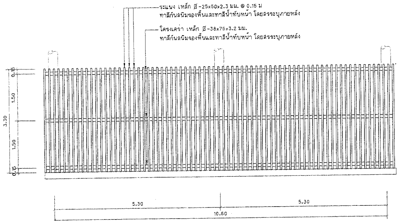
แปลนผนังตอกแต่งบริเวณสนามเด็กเล่น SCALE 1:50
