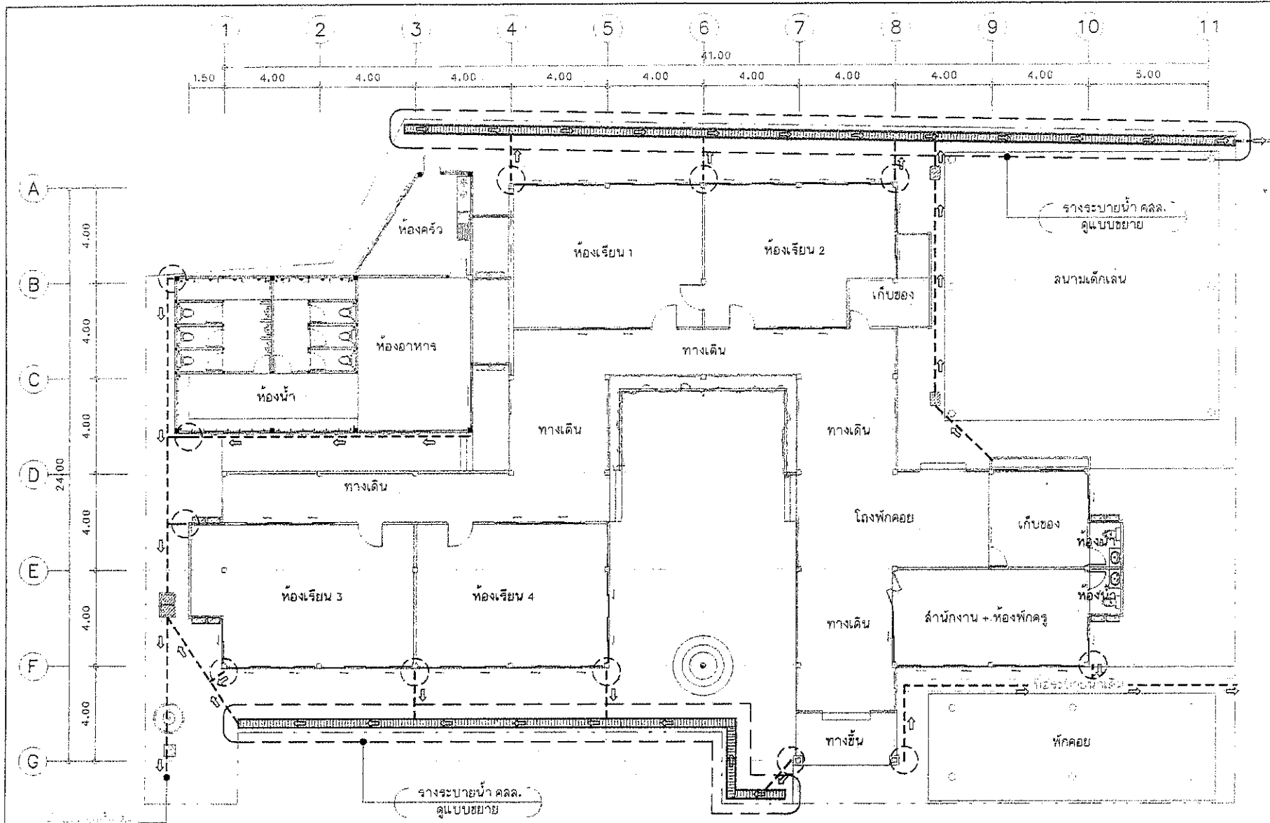
แปลนปรับปรุงระบบระบายน้ำ SCALE 1:150
