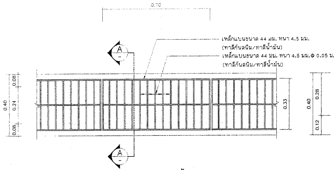
แบบขยายจางระบายน้ำ คสล. SCALE 1:10
