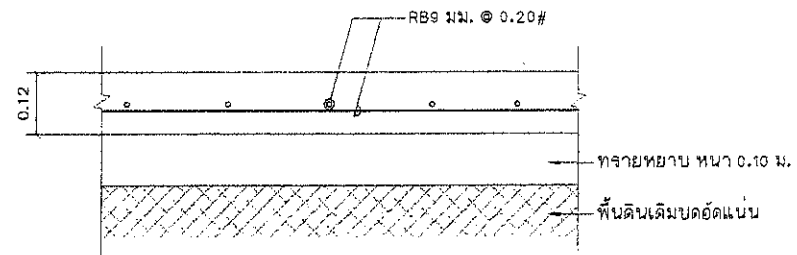
แบบขยายโครงสร้างพื้นอาคาร SCALE 1:10
