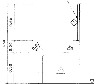
รูปด้าน (ข้าง) อ่างล้างมือ คสล. SCALE 1:20
