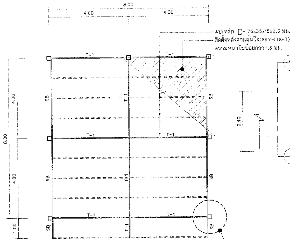
แบบขยายโครงหลังคา (ไปริ่งแลง) SCALE 1:75
