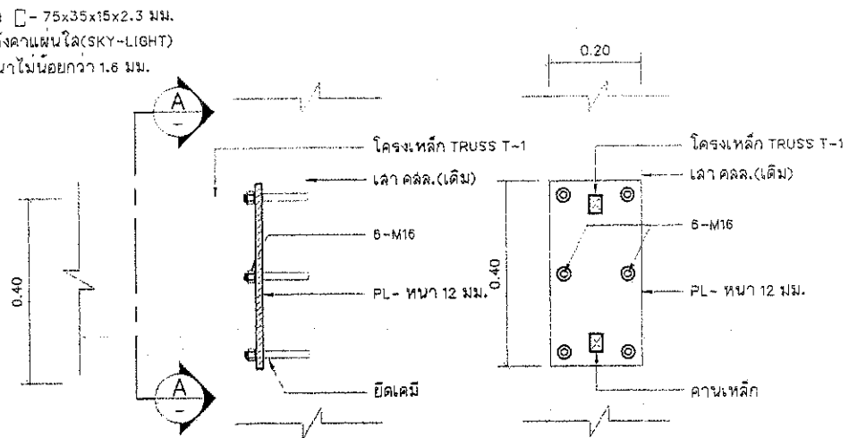
แบบขยายการติดตั้งโครงสร้างหลังคา SCALE 1:10
