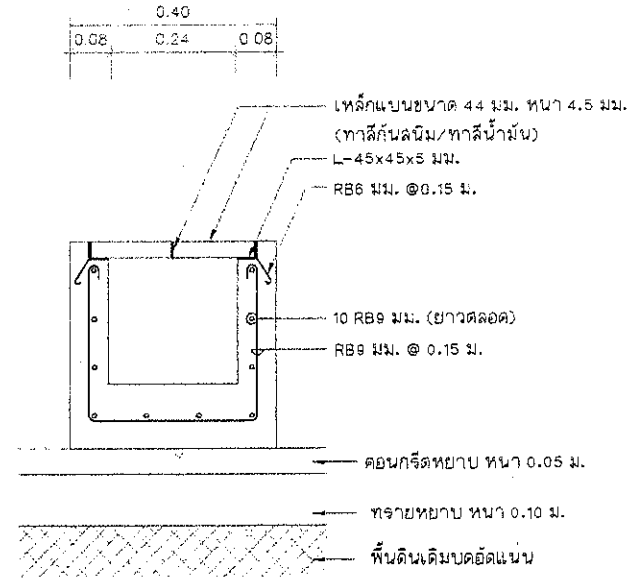
รูปตัด-A SCALE 1:10
