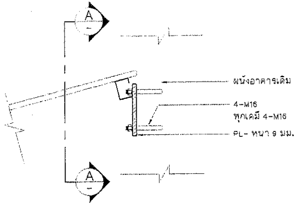
แบบขยาย โครงสร้างหลังค้ำด้านหลังอาคาร SCALE 1:10
