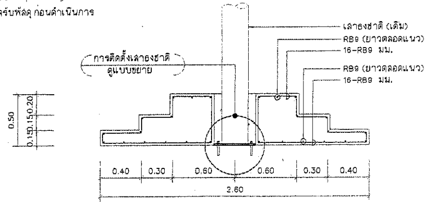
รูปตัด-A SCALE 1:25
