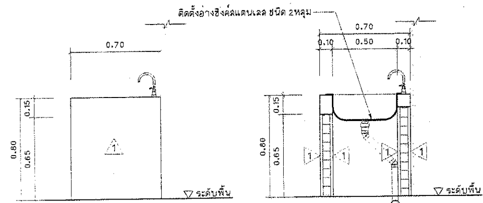
รูปด้าน (ข้าง) เคาน์เตอร์ล้างจาน SCALE 1:20
