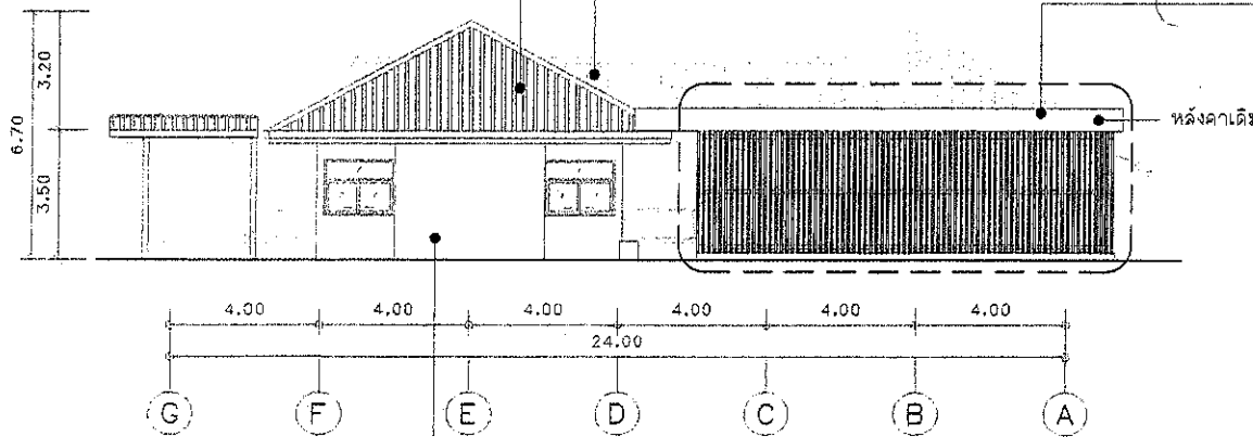
รูปด้าน-4 SCALE 1:150
