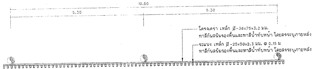
แปลนผนังตอกแต่งบริเวณสนามเด็กเล่น SCALE 1:50
