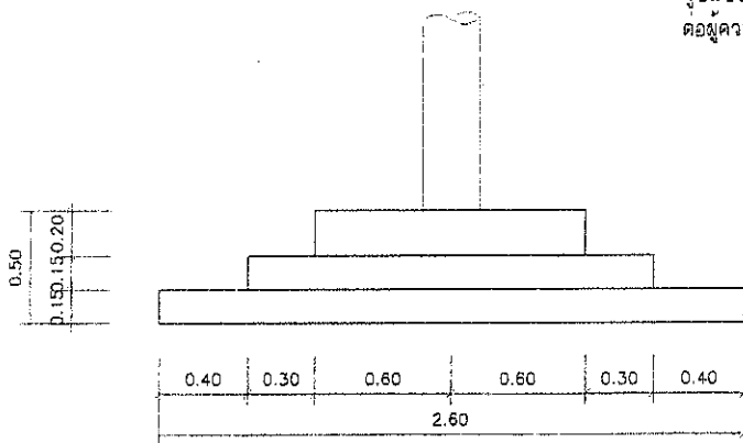
รูปด้าน (ฐานเสาธงชาติ) SCALE 1:25
