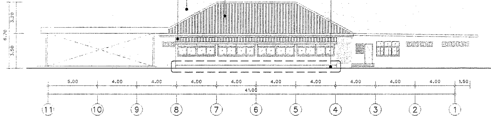
รูปด้าน-3 SCALE 1:150
