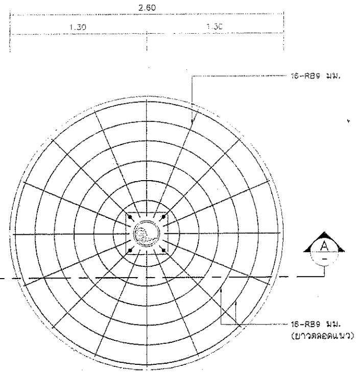
แปลนโครงสร้างฐานเสาธงชาติ SCALE 1:25
