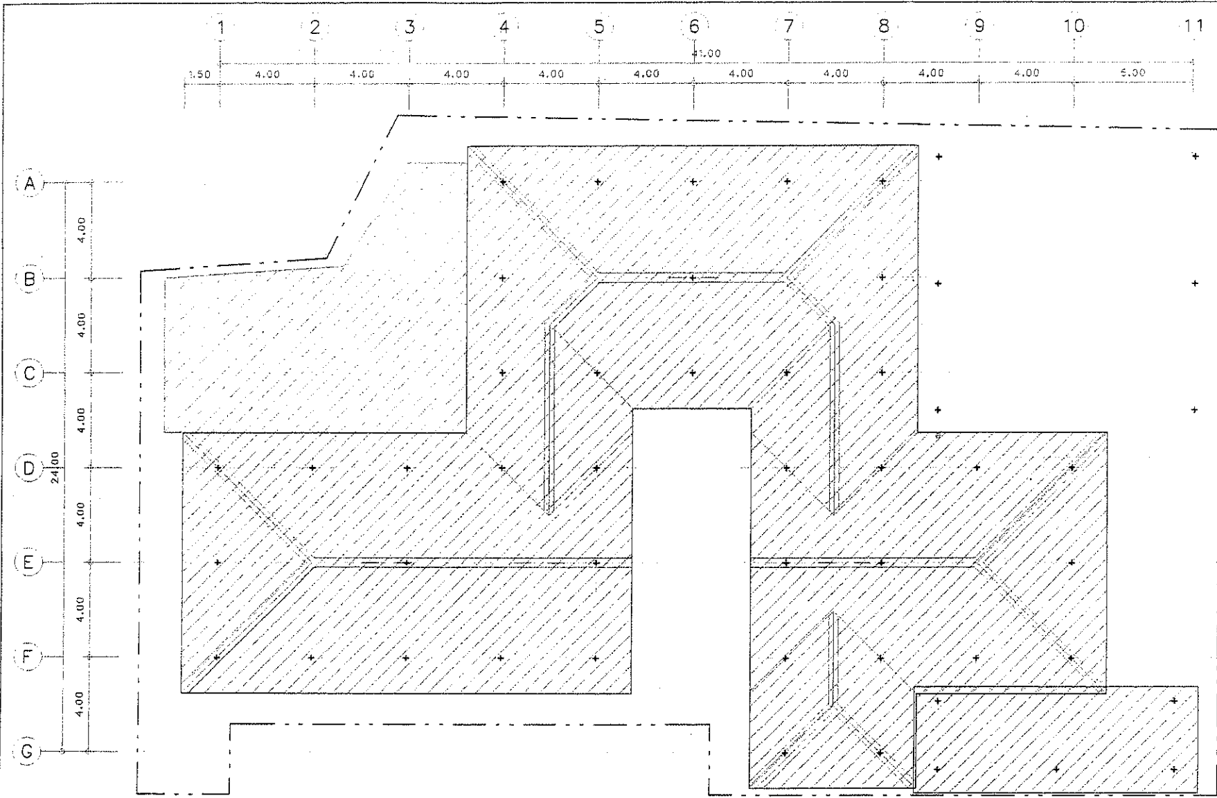
แปลนรื้อถอนหลังคาพร้อมโครงสร้างหลังคา SCALE 1:150
