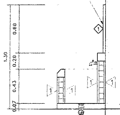
รูปตัด-A อ่างล้างมือ คสล. SCALE 1:20
