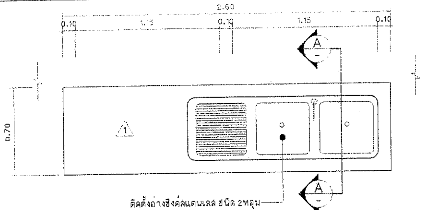
แปลนเคาน์เตอร์ล้างจาน SCALE 1:20
