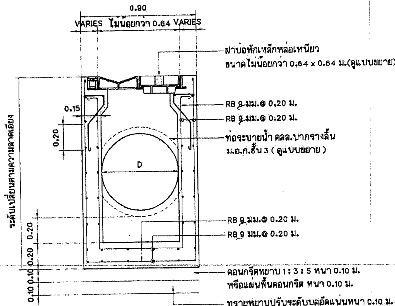
แบบขยายบ่อพัก คลอ. มาตราส่วน 1 : 20
