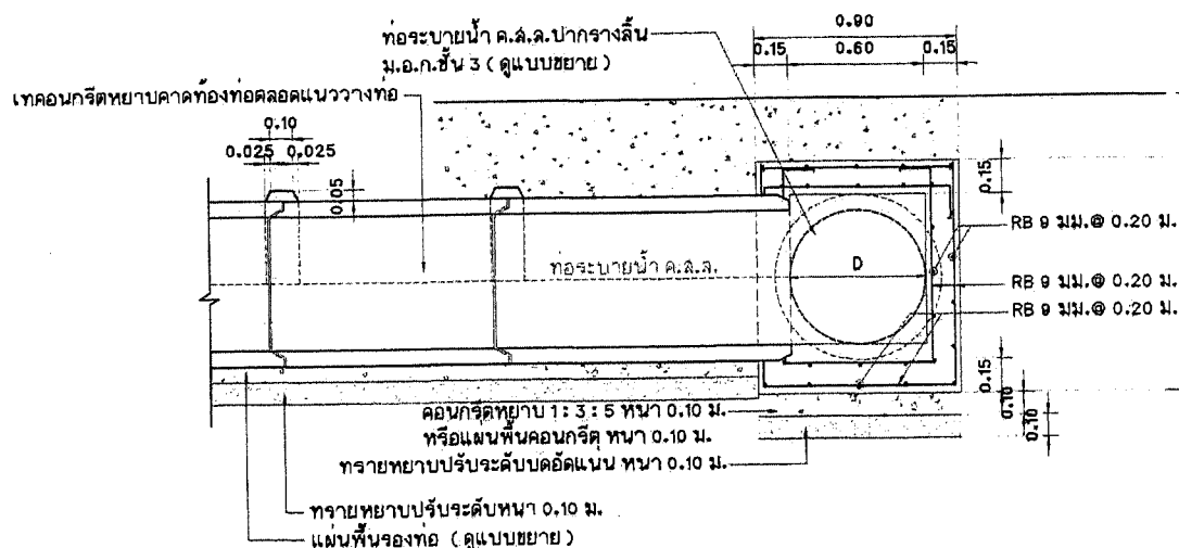
รูปตัดการเชื่อมต่อระบายน้ำของเดิม มาตราส่วน 1: 25
