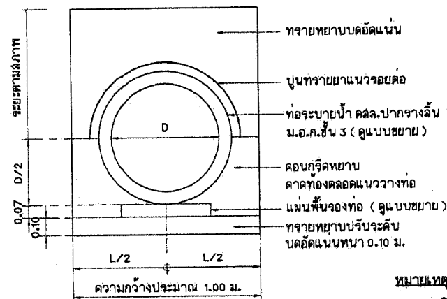
แบบขยายการวางท่อระบายน้ำ คลอ. มาตราส่วน 1 : 20
