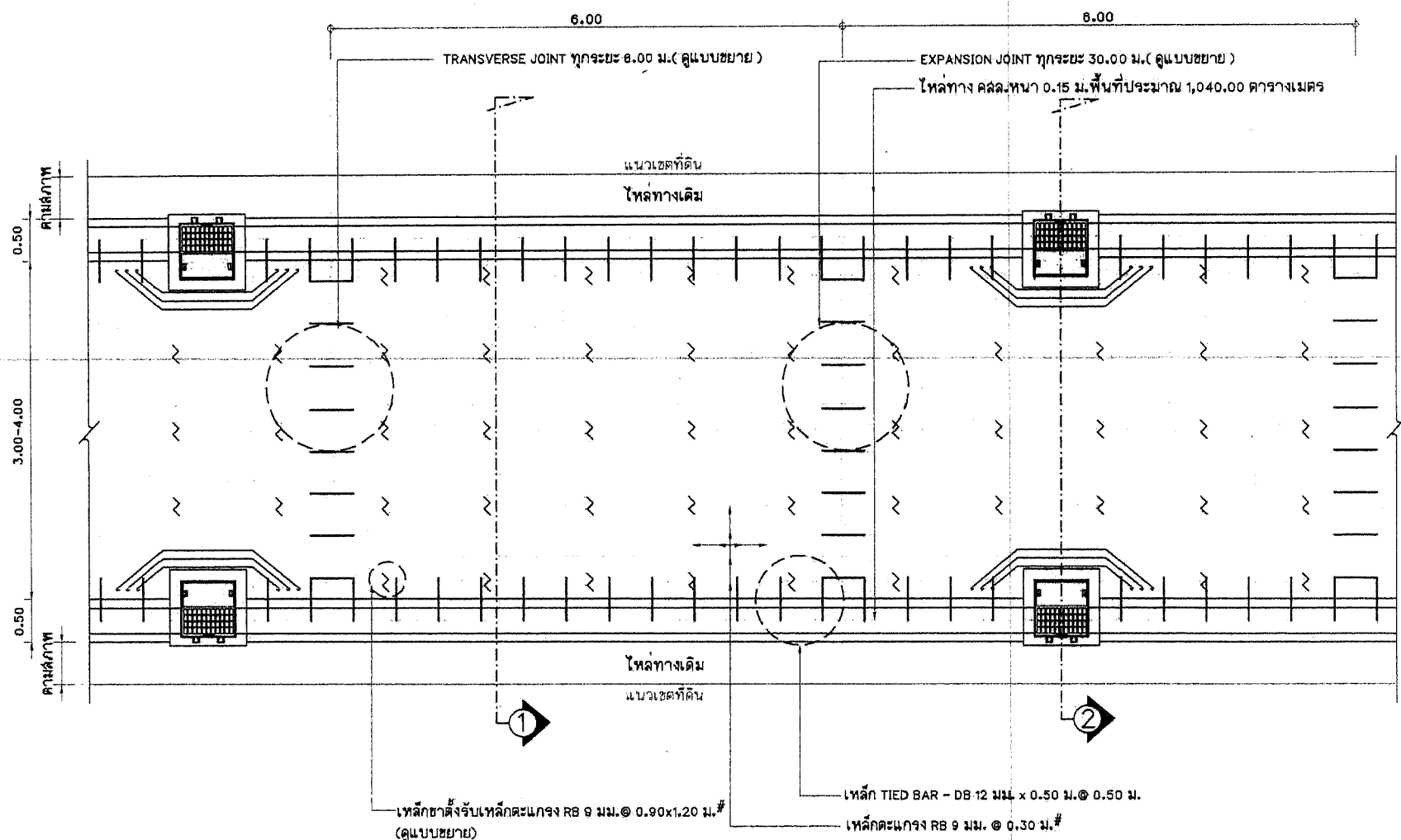
แปลนการวางเหล็กค้ำแรงและรอยต่อถนน คลล. มาตราส่วน 1 : 50
