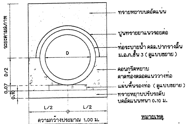
แบบขยายการวางท่อระบายน้ำ คล. มาตรฐาน 1:20
