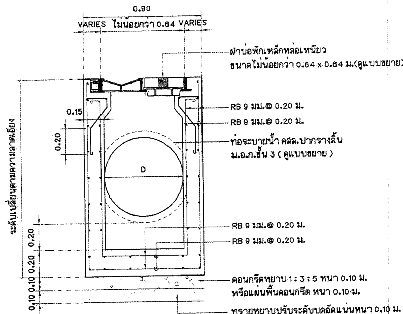
แบบขยายบ่อพัก คล. มาตรฐาน 1:20
