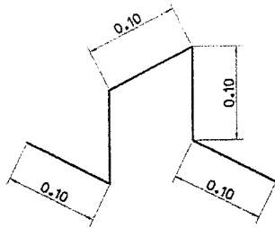
แบบขยายเหล็กขาตั้งรับเหล็กตะแกรง มาตรฐาน 1 : 5
