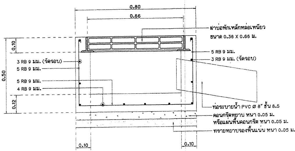
แบบขยายรูปตัด ② บ่อพักระบายน้ำ คลล. พร้อม ฝาบ่อพักรางวิ มาตราส่วน 1:10
