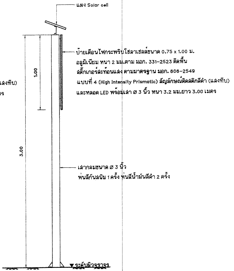
รูปด้านข้างป้ายเตือนไฟกระพริบโซล่าเซลล์ มาตรฐาน 1:20
