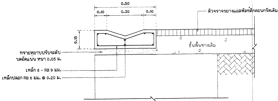
ขยายรูปตัดโครงสร้างรางระบายน้ำ ค.ส.ล. มาตราส่วน 1 : 10
