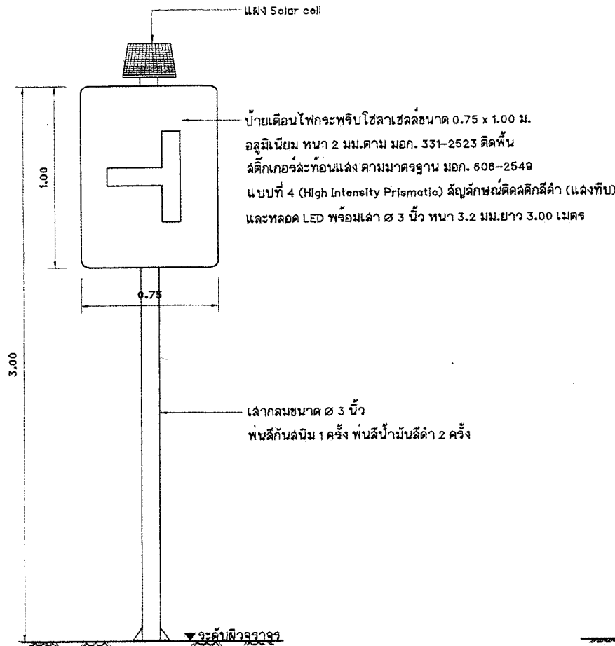
รูปด้านหน้าป้ายเตือนไฟกระพริบโซล่าเซลล์ มาตรฐาน 1:20
