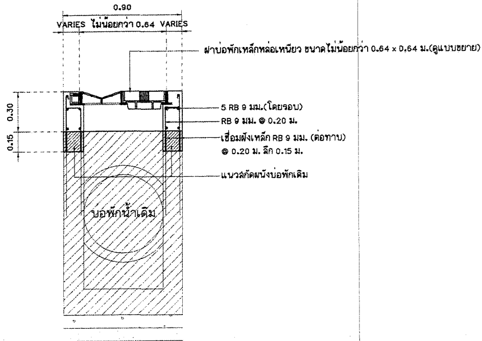
แบบขยายรูปตัดปรับปรุงขอบบ่อพัก ค.ส.ล.พร้อมฝาบ่อพักเหล็กหล่อเหนียว มาตราส่วน 1 : 20
