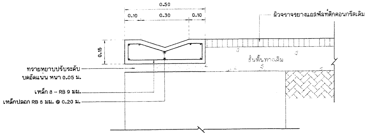
ขยายรูปตัดโครงสร้างรางระบายน้ำ ค.ล.ล. มาตราส่วน 1 : 10
