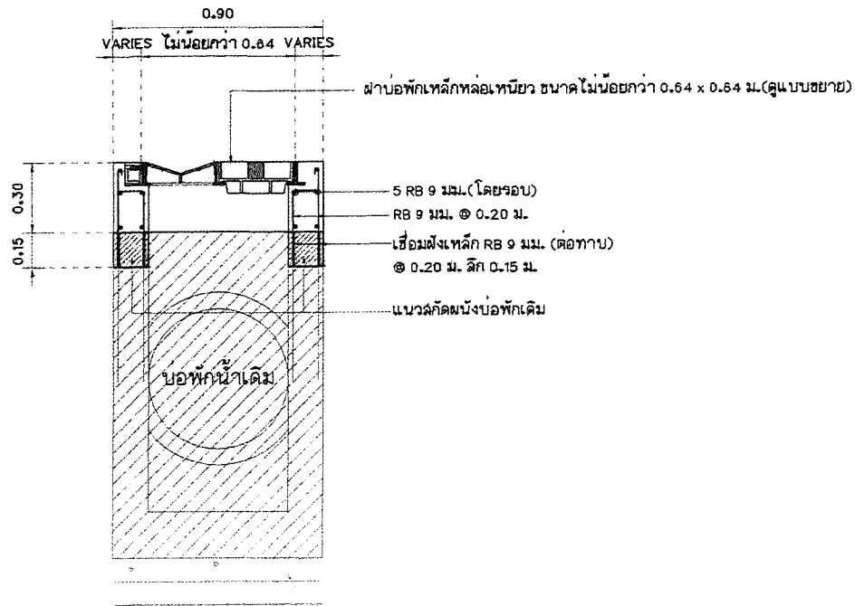
แบบขยายรูปตัดปรับปรุงขอบบ่อพัก ค.ล.ล. พร้อมฝาบ่อพักเหล็กหล่อเหนียว มาตราส่วน 1 : 20
