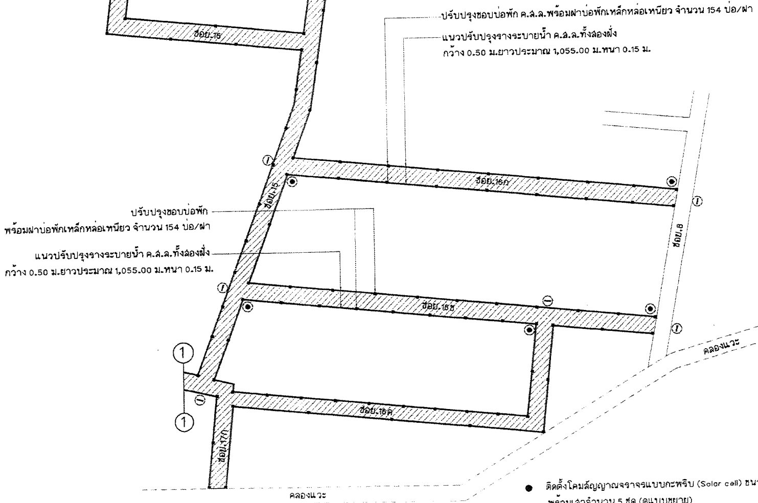
แปลนปรับปรุงรางระบายน้ำพร้อมฝาบ่อพัก มาตรฐาน 1 : 1000
