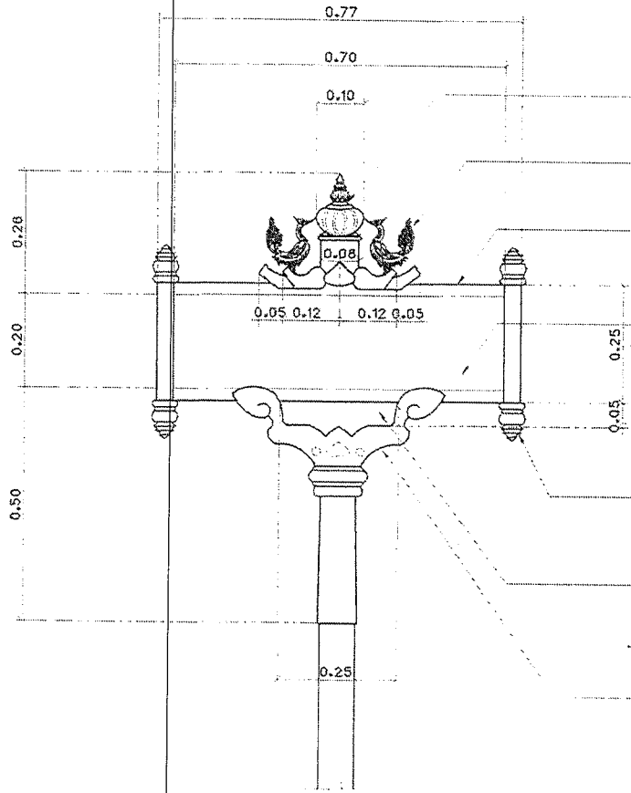
แบบขยายป้าย ด้านหน้า - หลัง มาตราส่วน 1 : 10
