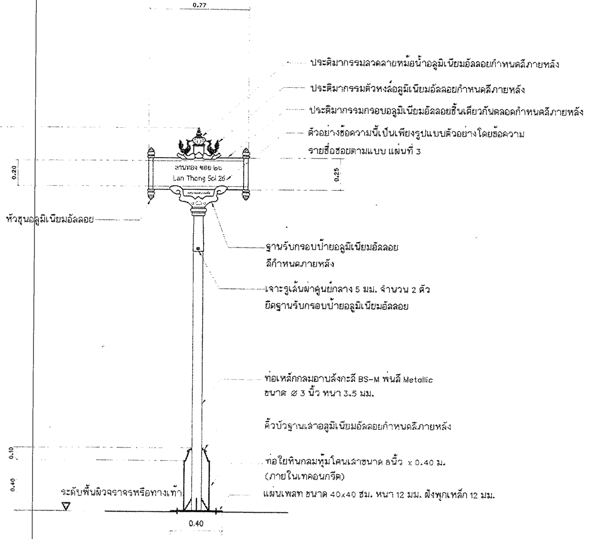
รูปตัดการติดตั้งป้าย (แบบที่ 2) มาตราส่วน 1 : 20
