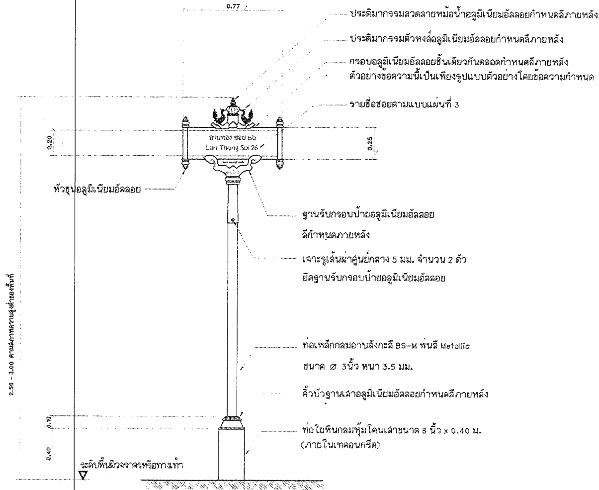
รูปด้านหน้า - หลัง (ป้ายบอกชื่อซอยและเสา) มาตรฐาน 1 : 20
