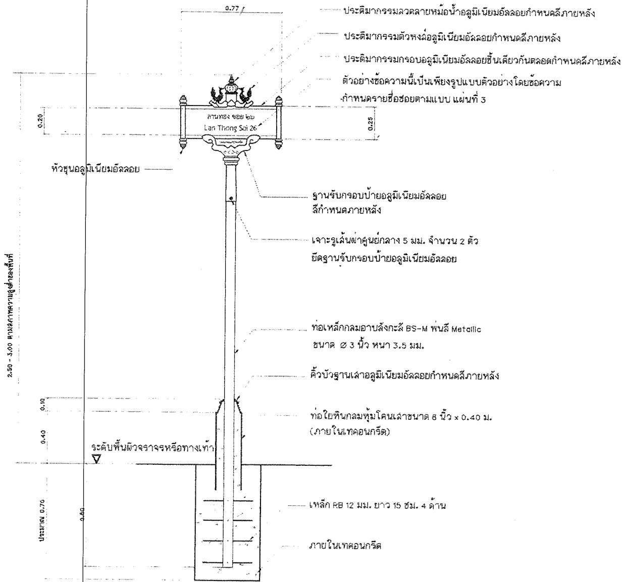
รูปตัดการติดตั้งป้าย (แบบที่ 1) มาตราส่วน 1 : 20
