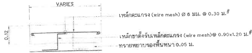
แบบขยายรูปตัดไหลทาง และ ทางเข้าบ้าน คสล.หนา 0.12 ม. มาตรฐาน 1 : 10
