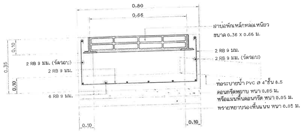
แบบขยายรูปตัด ② บ่อพักระบายน้ำ คลล. พร้อม ฝาบ่อพักรางวี มาตราส่วน 1 : 10
