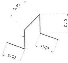
แบบขยายเหล็กขาตั้งรับเหล็กตะแกรง (ไหลทาง คสล.หนา 0.12 ม.) มาตรฐานควบคุมกำหนด
