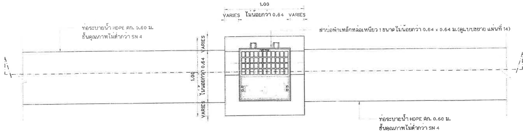
แปลนการวางท่อระบายน้ำ
