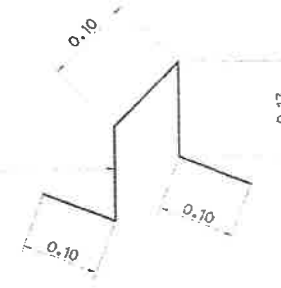
แบบขยายเหล็กขาตั้งรับเหล็กตะแกรง (ผิวถนนคสล.หนา 0.15 ม.) มาตรฐานตามกำหนด
