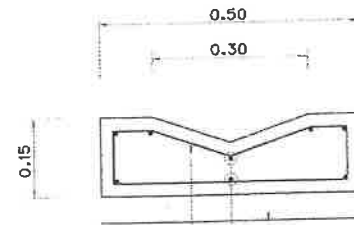
แบบขยายรูปตัดไหลทาง และ ทางเข้าบ้าน คสล.หนา 0.12 ม. มาตรฐาน 1 : 10
