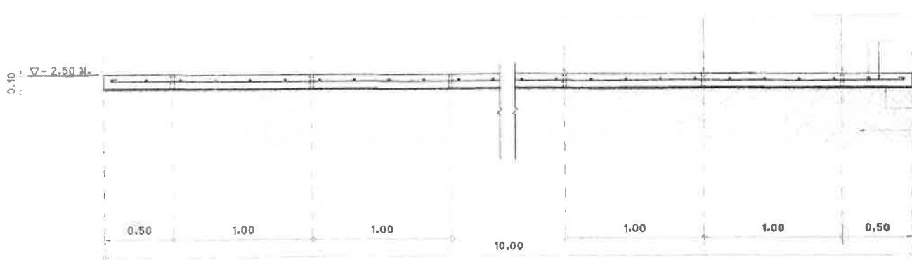
รูปตัดดาดท้องคลอง มาตราส่วน 1:25
