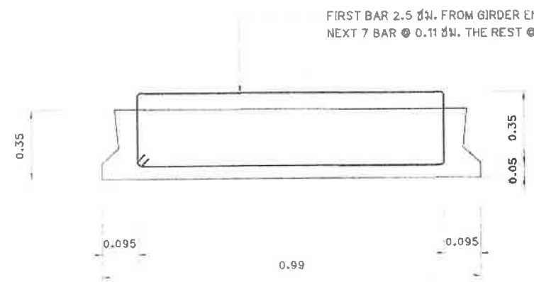
PLANK 10.00 ม. SPAN
