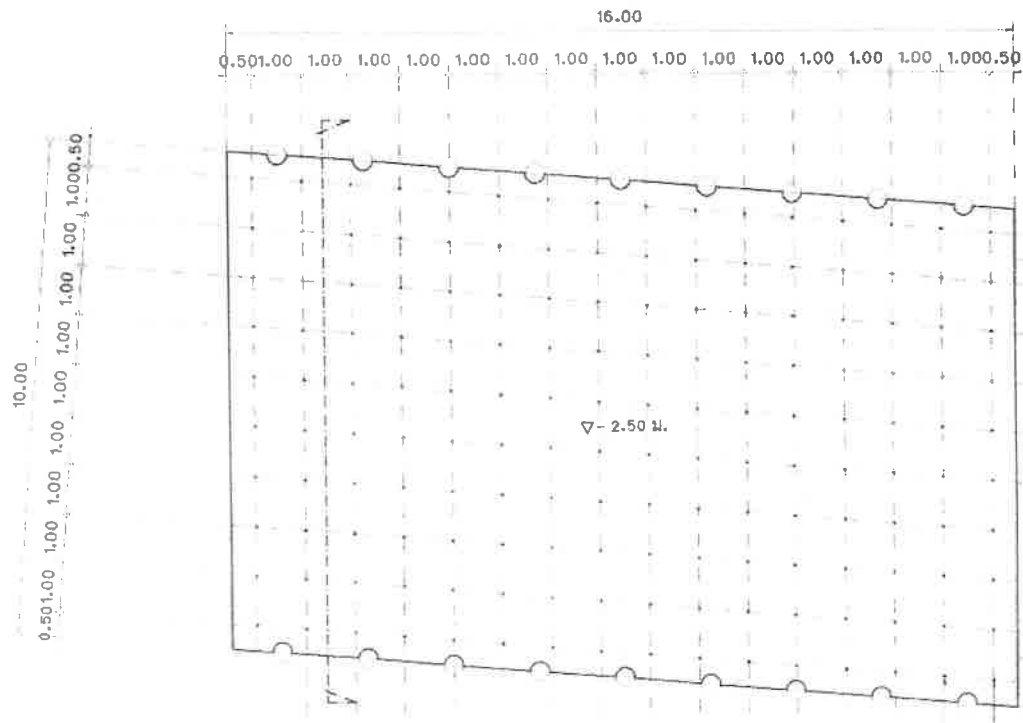
แปลนเสาเข็มดาดท้องคลอง มาตราส่วน 1:100
