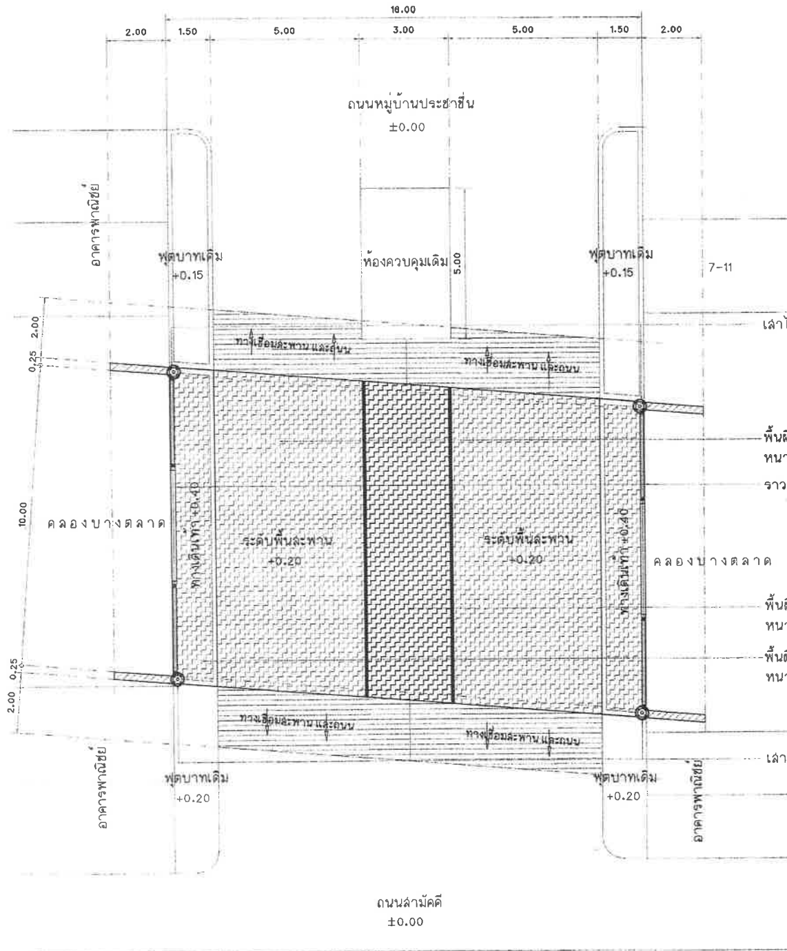
แปลนพื้นสะพาน คสล.บริเวณหมู่บ้านประชาชน มาตรฐาน 1:125
