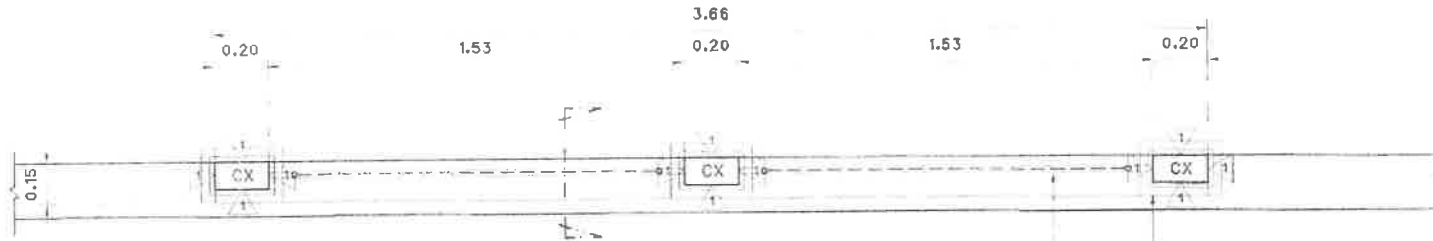
แบบขยายแปลนโครงลวดราวสะพาน คลล. มาตราส่วน 1:20
