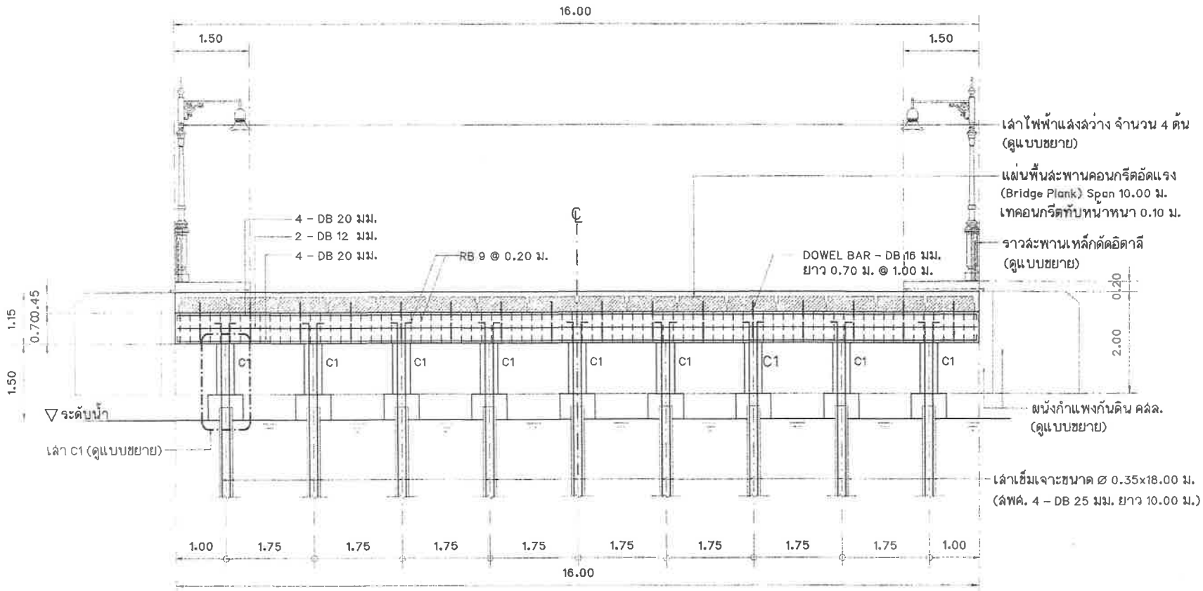
รูปตัดโครงสร้างสะพาน A - A
