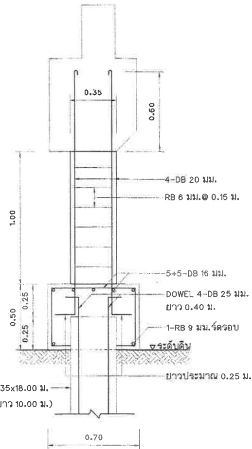
รูปตัดเส้า C1
