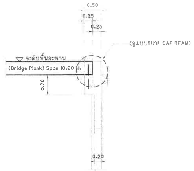
CAP BEAM มาตราส่วน 1:50
