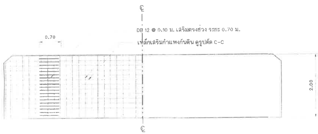
แบบขยายกำแพงกันดิน มาตราส่วน 1:50
